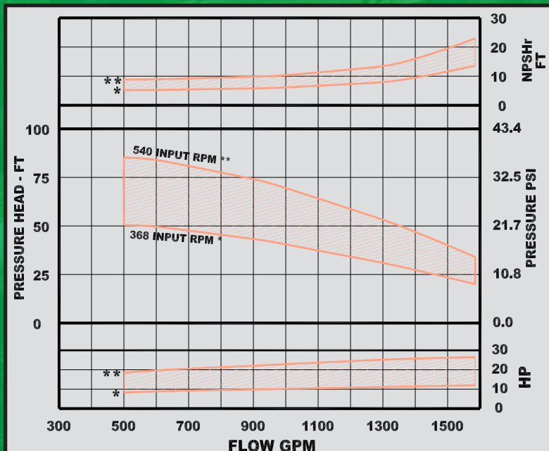
PTO Input - 540 RPM
